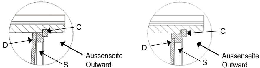
Sicherungsring S Variante 1 und 2 - Korrekte Montage Locking ring S , type 1 and 2 - Proper placement
